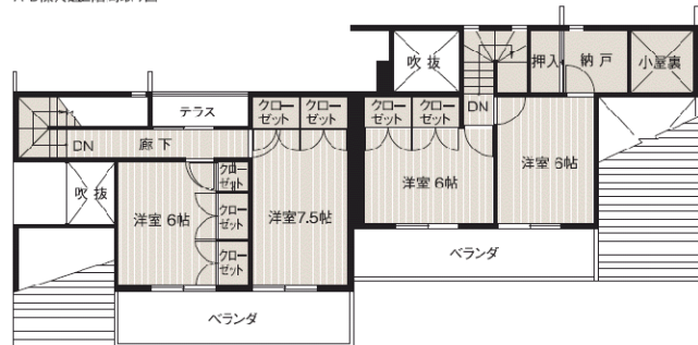
A・B楼共通2階間取り図
